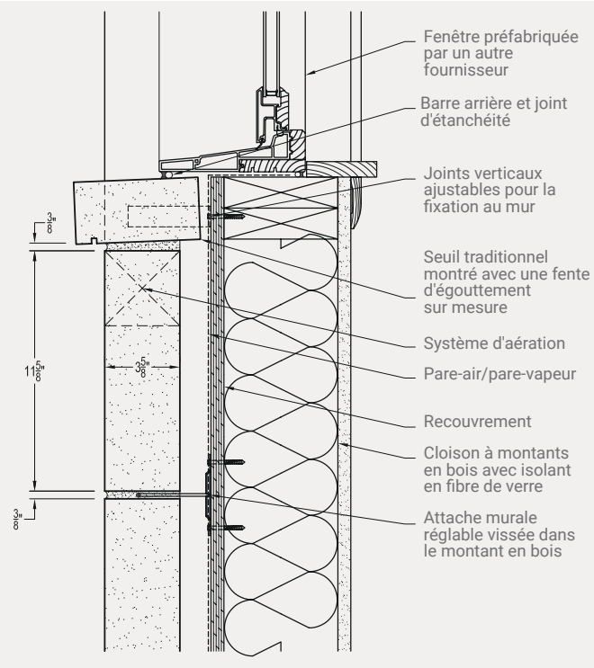
SCHÉMA DE L'INSTALLATION D'UN SEUIL DE FENÊTRE
