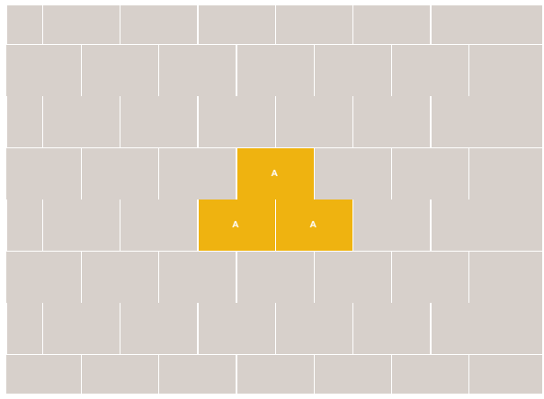
VANDERBILT CLASSIC™ - APPAREIL EN PANNERESSE (16 x 24)
