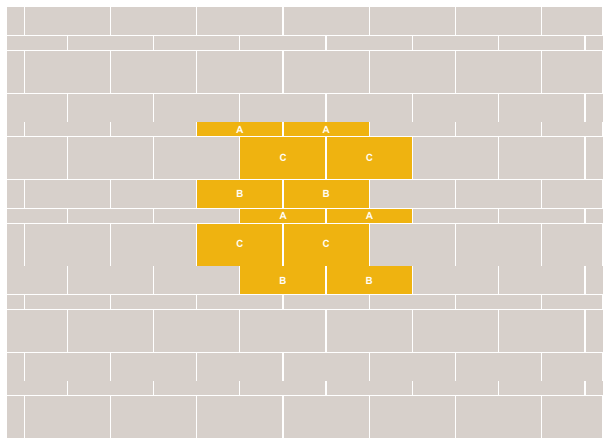
VANDERBILT CLASSIC™ - APPAREIL EN PANNERESSE 3 MODULES
